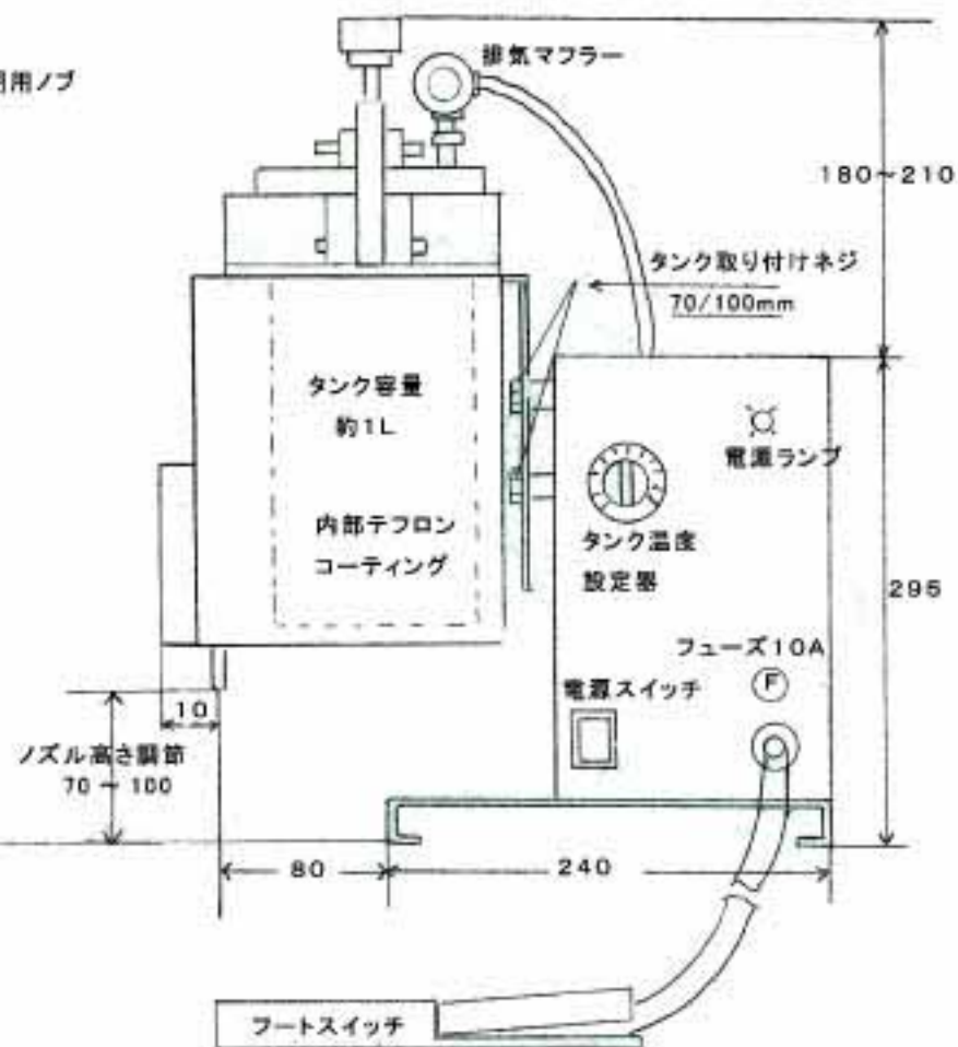
側面図
