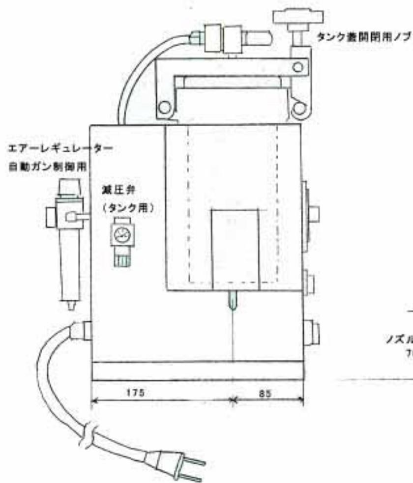
正面図
